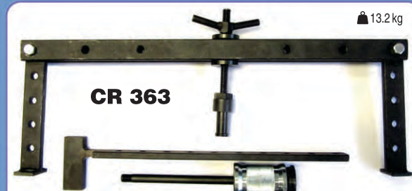
CR 363 Dispositivos para retirar bico injetor eletrônico. Carretel Rosca M27 X 1mm. Sistema (sacador com rosca) em linha, ou individual no sistema (à percussão) Acompanha adaptador para Renault Master (apoiar na caixa seca do câmbio). OBS: Os bicos devem ser de rosca M27 X 1mm e estar sem o solenóide, em condições normais.
