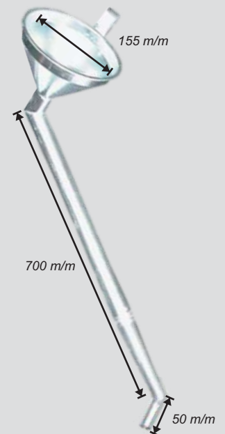
Funil Kombi (LUB-56)
