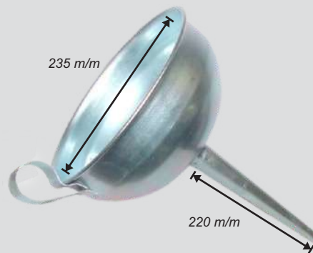
Funil uso geral grande (LUB-55C)
